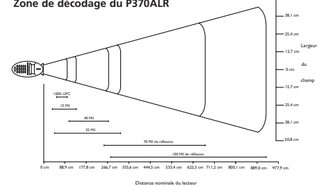
Zone de décodage du P370ALR
