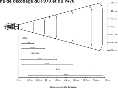
Zone de décodage du P370 et du P470
